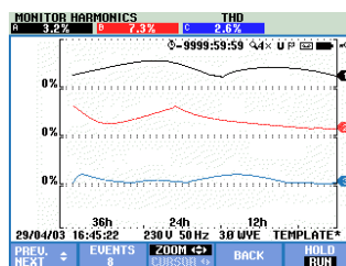
Рис. 16-2 Дисплей трендов
