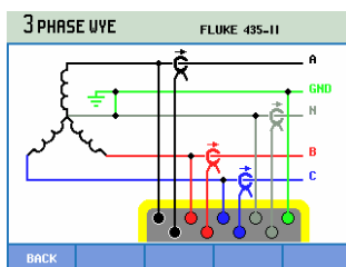
Рис. 24-3 Экран с действующей конфигурацией проводки
