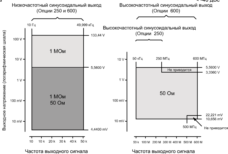
Синусоидальный выход - высочастотные и низкочастотные характеристики "напряжение - частота"
